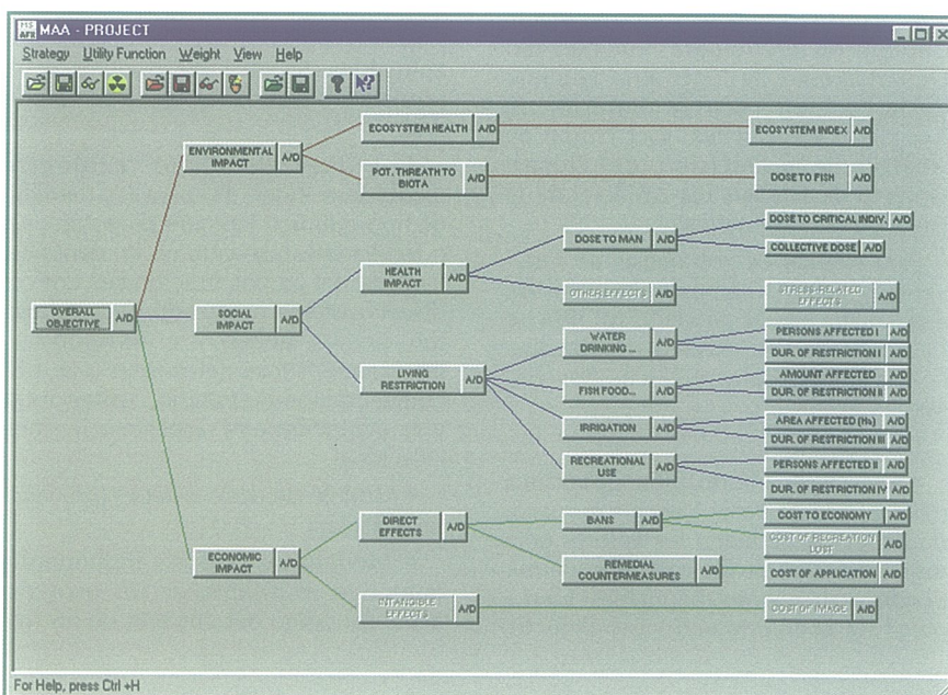
Figura 2.- Árbol de objetivos considerados para el Análisis de utilidad Multi-Atributos en el sistema MOIRA.
