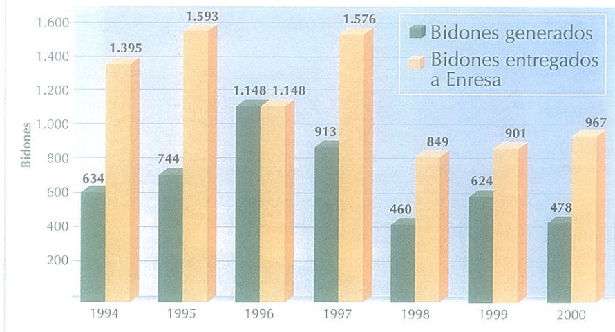
Sta. M a de Garoña. Generación de residuos de baja y media actividad 1994 - 2000
