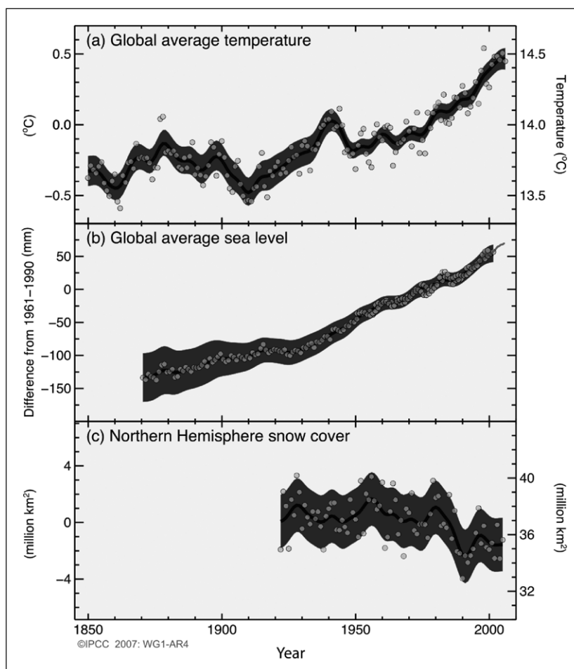
Figura 1. Evolución de los valores medios de temperatura, nivel del mar, y superficie cubierta de nieve (en el hemisferio norte). Se toma como valor de referencia la media del periodo 1961-1990. (Fuente: 4º Informe IPCC)
