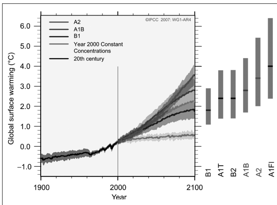
Figura 3. Las curvas representan la evolución futura de la temperatura estimada para los distintos escenarios estudiados por el IPCC. A la derecha de incluyen los intervalos de incertidumbre. Las mayores temperaturas se producen para las emisiones más altas de gases invernadero. En el escenario peor a finales del siglo XXI se producirían incrementos de temperatura de hasta 6 °C mayores que las actuales. Se da la circunstancia que la situación presente corresponde a los escenarios más pesimistas de informes pasados del IPCC. (Fuente: 4º Informe IPCC)
