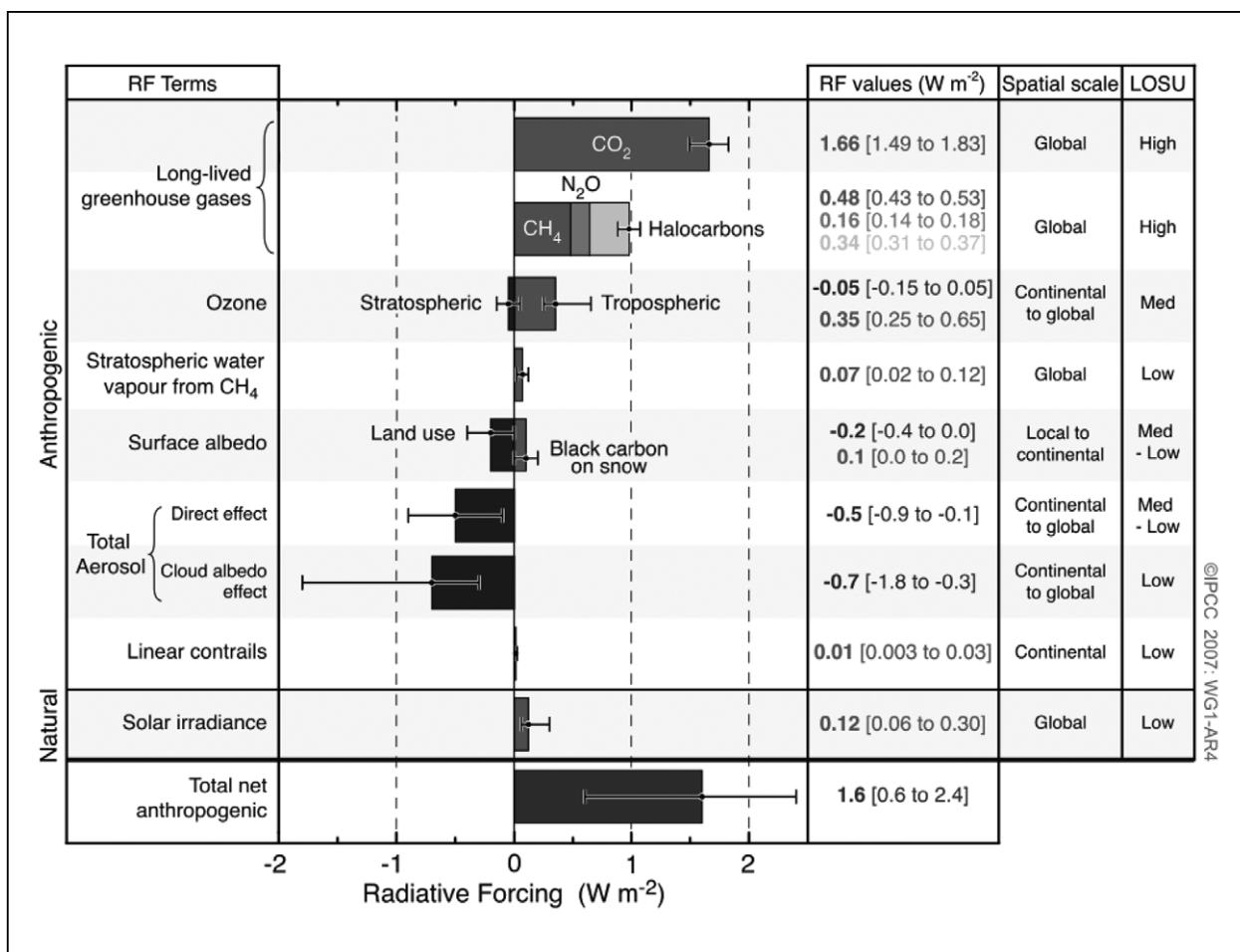
Figura 2. Reforzamiento radiativo (RF) actual para los factores más significativos que inciden en el balance energético. Se incluye los intervalos de confianza calculados con un 90% de incertidumbre. El balance neto promedio es 1.6 W/m 2 , que corresponde al calor que queda atrapado en el planeta. (Fuente: 4º Informe IPCC)
