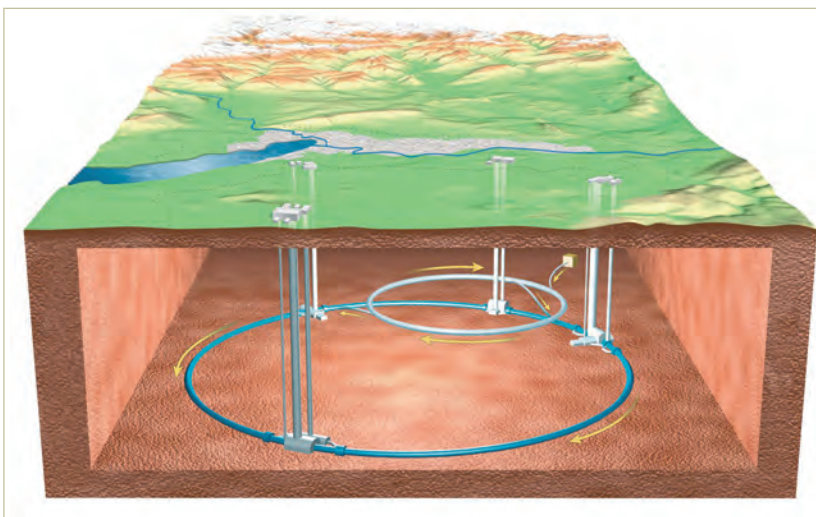
Figura 2. Una visión general del LHC. Fuente CERN.
