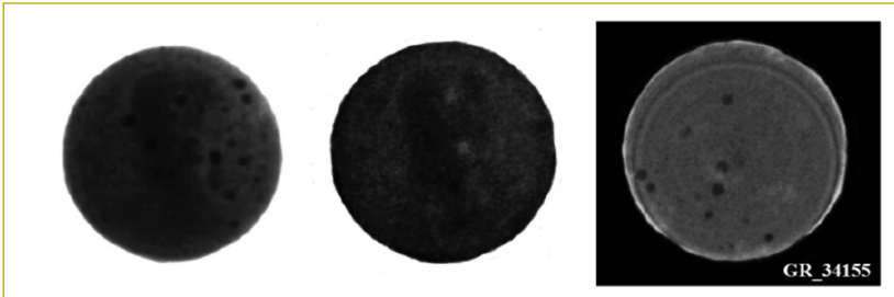
Figura 4: Imagen de una moneda de cobre de la Grecia clásica mediante rayos X (izquierda) y neutrones (centro y derecha) [2].
