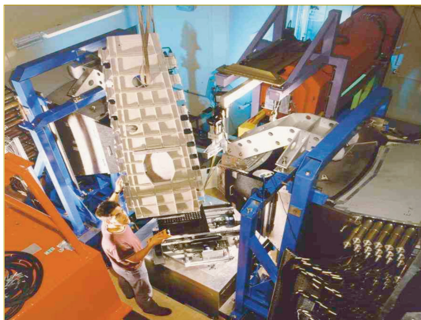
Figura 7: Posicionamiento de una pieza de Airbus en el instrumento ENGIN-X de la fuente ISIS.
