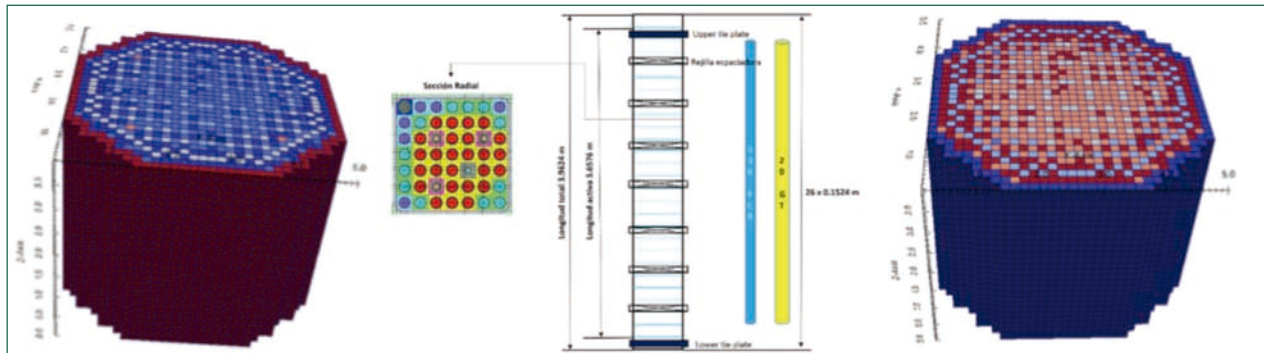
Figura 9. Esquema del modelo de CTF y Parcs del núcleo del reactor de Peach Bottom Unit 2.
