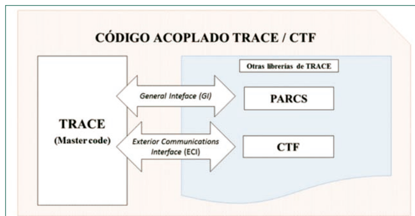
Figura 1. Esquema del código acoplado TRACE/CTF.
